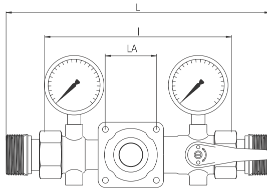
Flange
